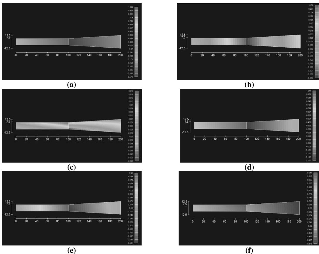
Gambar 3. Kontur Tegangan: (a) Tegangan Normal x ; (b) Tegangan Normal y ; (c) Tegangan Geser xy ; (d) Tegangan Maksimum; (e) Tegangan Minimum; (f) Tegangan Von Mises
