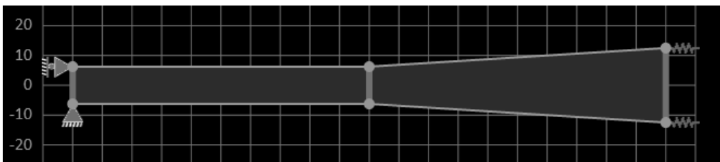
Gambar 7. Material Orthotropik dengan Q4, Plane Stress
