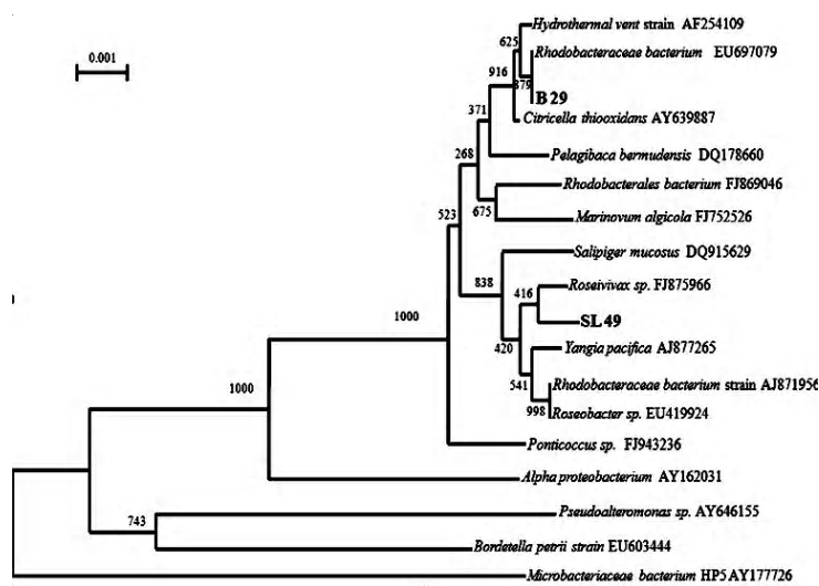
Gambar 5. Pohon kekerabatan 2 bakteri potensial pendegradasi phenanthrene yaitu B29 ( Rhodobacteraceae bacterium F9) dan bakteri SL49 ( Roseobacter sp. RW 37) dengan kelompok luar sebagai pembandingan Microbacteriaceae bacterium yang dianalisis dengan program BioEdit . Tingkat ketelitian dendrogram ditentukan melalui nilai bootstrap dengan pengulangan 1000 kali.
