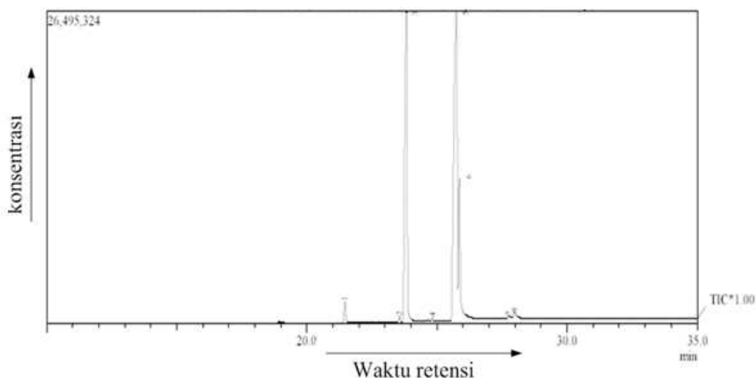
Gambar 1. GS-MS Metil ester Campuran Minyak Sapi dan Minyak Sawit
