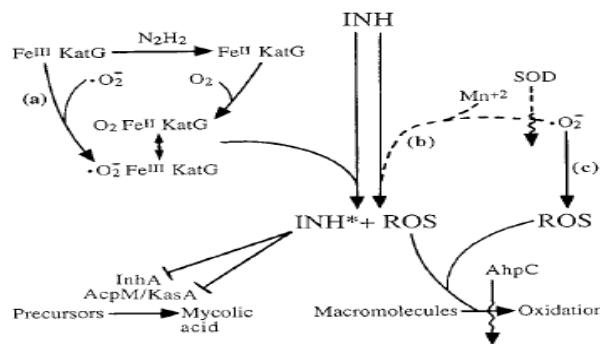
Gambar 4. Potensi keterlibatan superoksida dalam aktivitas INH . INH sebagai prodrug yang diaktivkan oleh protein KatG (katalase - peroksidase) atau oleh Mn 2+ . Di sebelah kiri gambar adalah skema yang menunjukkan bentuk KatG non-aktif (Fe III KatG) yang diubah menjadi bentuk aktif oleh dua jalur, salah satunya (a) membutuhkan superoksida (O 2 - ). Di sebelah kanan adalah skema yang menunjukkan aktivasi INH oleh jalur dependen Mn 2+ yang juga melibatkan superoksida (b), jalur ini dapat dihambat oleh superoksida dismutase (SOD). Jalur ini ditunjukkan dengan garis putus-putus karena mungkin tidak signifikan secara in vivo. INH aktif (INH*) menghambat sintesis asam mikolat dengan cara menonaktifkan InhA dan ACPM - KasA . Spesies oksigen reaktif (ROS) timbul selama aktivasi INH atau akibat kehadiran superoksida (c). Protein AhpC muncul untuk membatasi akumulasi kerusakan oksidatif makromolekul yang diharapkan timbul dari aktivasi INH atau adanya superoksida. Garis bergelombang menunjukkan penghambatan jalur, dan jalur dengan bar tegak lurus menunjukkan penghambatan enzim. 40
