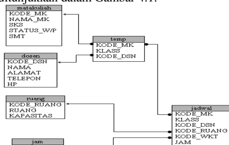
Gambar 4.1 E-R Diagram Sumber : Perancangan Sistem Gambar 4.1. ER Diagram
