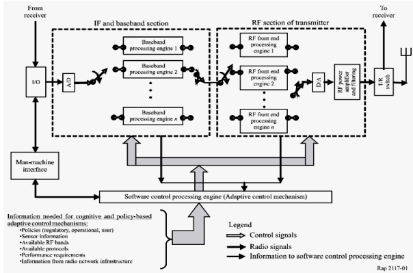
Gambar 1. Arsitektur SDR [6].
