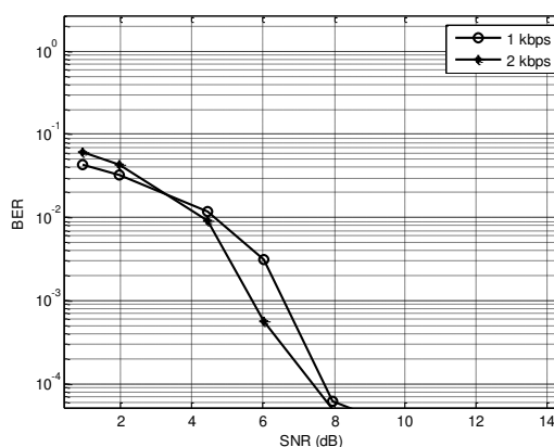
Gambar 5. Grafik BER vs SNR Sistem Modem dengan Simulasi.
