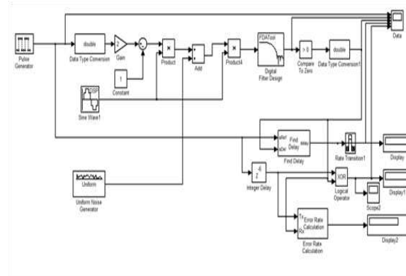
Gambar 4. Diagram Blok Simulasi Modem.
