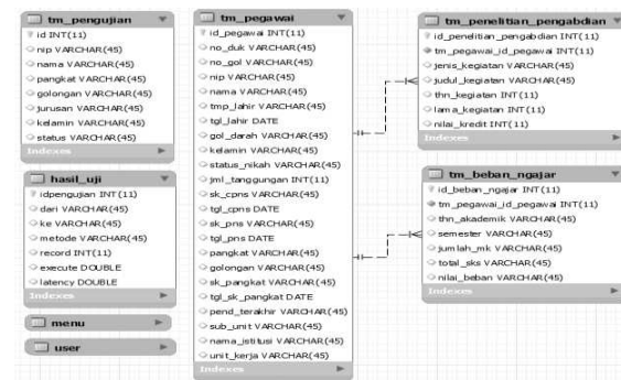
Gambar. 11. Basis Data Aplikasi Kepegawaian
