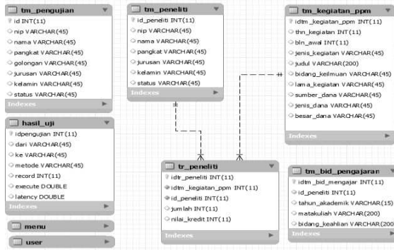
Gambar. 12. Basis Data Aplikasi Penelitian
