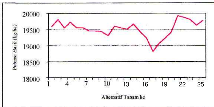
Gambar 4. Fluktuasi potensi hasil selama satu tahun berdasarkan hasil simulasi masa tanam dua mingguan
