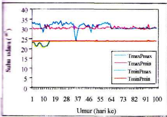
Gambar 1. Embutan suhu udara maksimum dan minimum da lain kondisi potensi hasil lertiaggi dan tercnadah.
