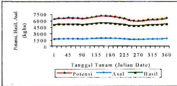
Ciambar 3. Asal, Hasil dan Potensi berdasarkan hasil simulasi tanggal tanam 2 iningguan
