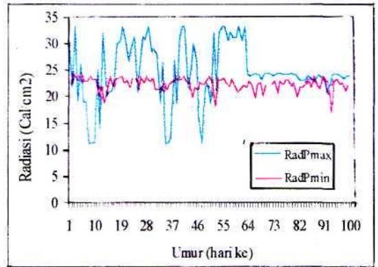
(Jambar 2. Embutan radiasi pada potensi hasil fertinggi dan tercnadah
