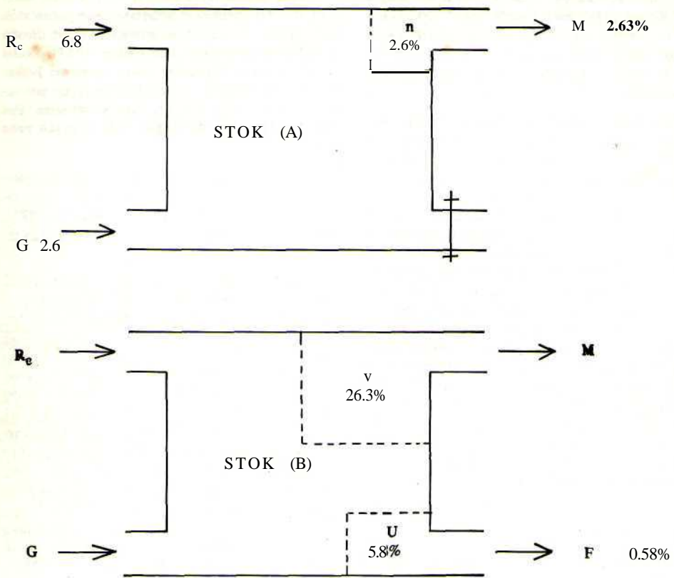
Gambar 2. Diagram dinamika stok S mossam-Metis di Waduk Selorejo, pada saat tidak ada penangkapan (A) dan pada saat ada penangkapan (B). • - ' ; Vs:- • R_c : laju peremajaan, n : laju mortalitas alami yang terjadi bila tidak ada mortalitas penangkapan, v : laju mortalitas alami yang dihapalkan ter-
