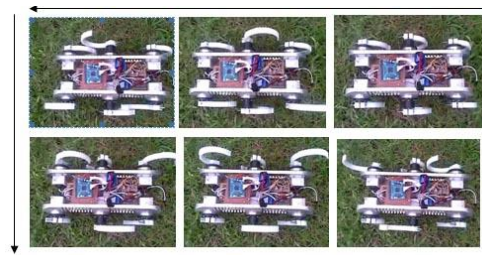
Gambar 19. Pengujian Pergerakan Maju Robot
