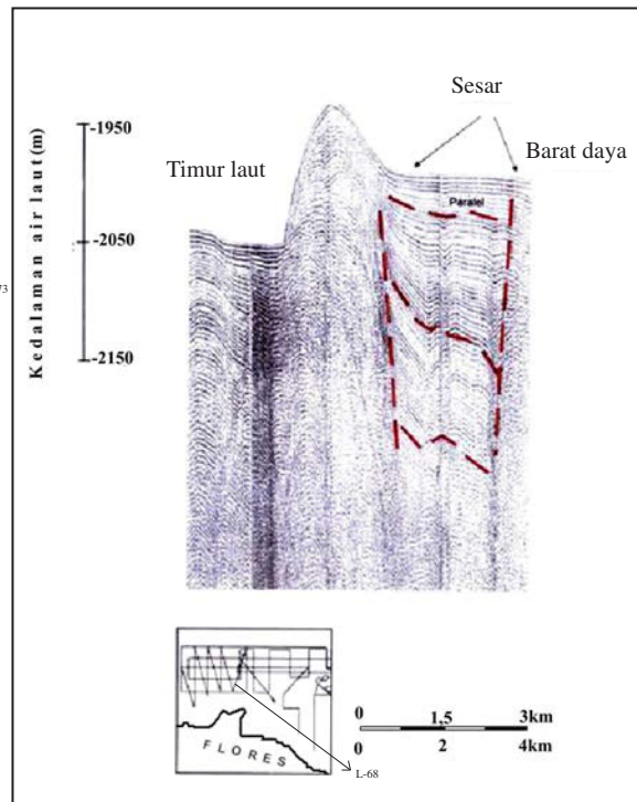
Gambar 7. Rekaman seismik pantul L-68.
