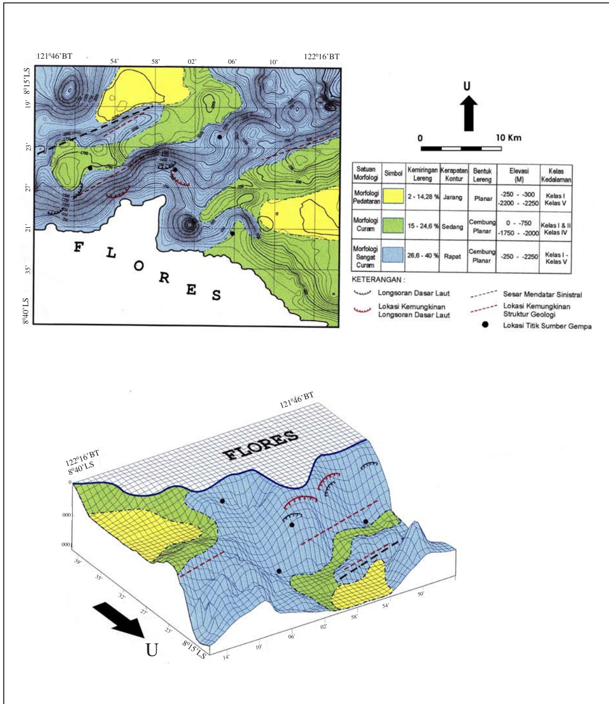
Gambar 10. Peta dan blok diagram struktur geologi dan longsor bawah laut, perairan Flores, Nusa Tenggara Timur.
