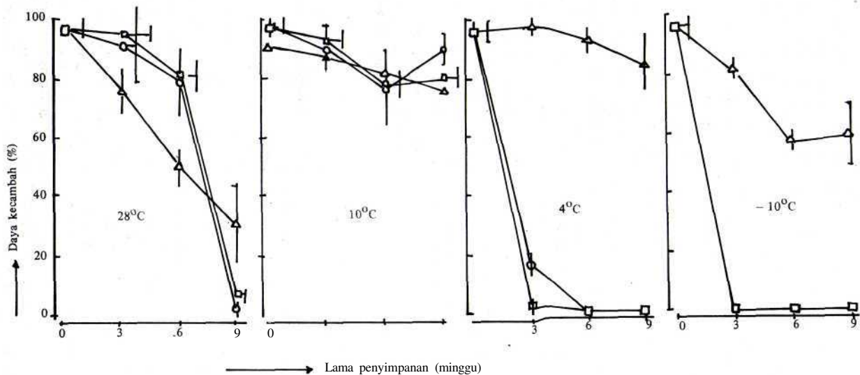
Gambar 2. Daya kecambah biji kemuning ( M. pankulata ) setelah disimpan selama 9 minggu pada berbagai suhu dan kadar air (0 - 24,1 5% ; • = 16,7%; ▲ = 5,0%). Garis vertikal menunjukkan simpangan bakunya.
