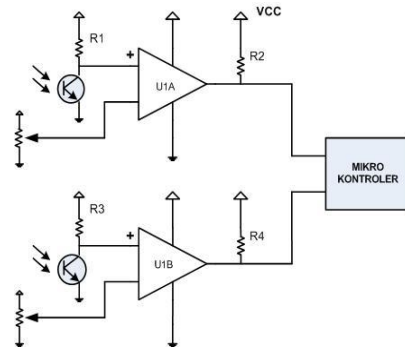
Gambar 3. Skema Rangkaian Sensor Infra Merah
