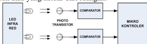
Gambar 2. Blok Diagram Sensor Infra merah
