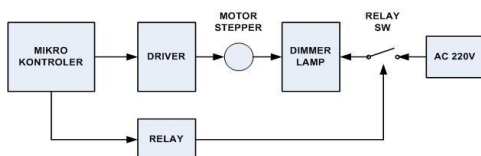
Gambar 5. Blok Diagram Pengaturan Rangkaian Dimmer
