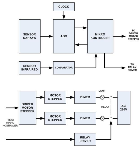
Gambar 6. Diagram Blok Rangkaian Pengatur Lampu Otomatis
