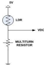
Gambar 1. Rangkaian Sensor Cahaya
