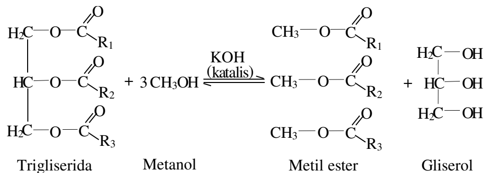
Gambar 2. Reaksi transesterifikasi trigliserida menggunakan metanol
