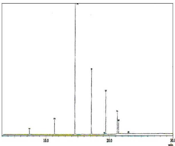
Gambar 3. Kromatogram biodiesel dari minyak goreng bekas
