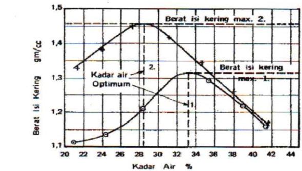
Gambar 2. Pengaruh kadar air dan usaha pemadatan terhadap kepadatan tanah
