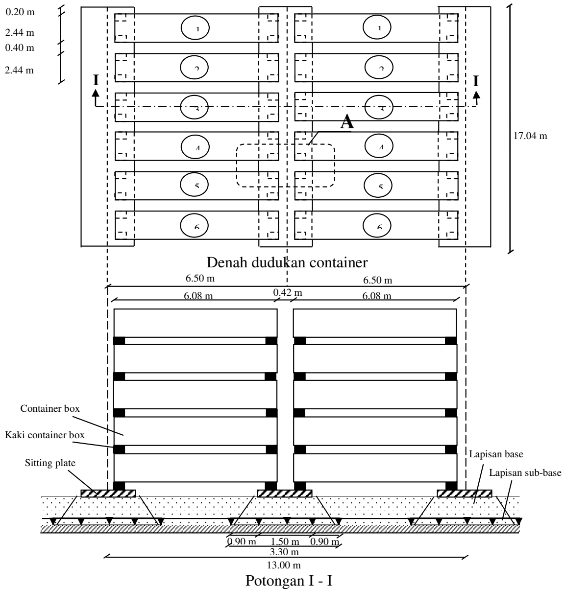
Gambar 5 Beban yang bekerja akibat tumpukan peti kemas
