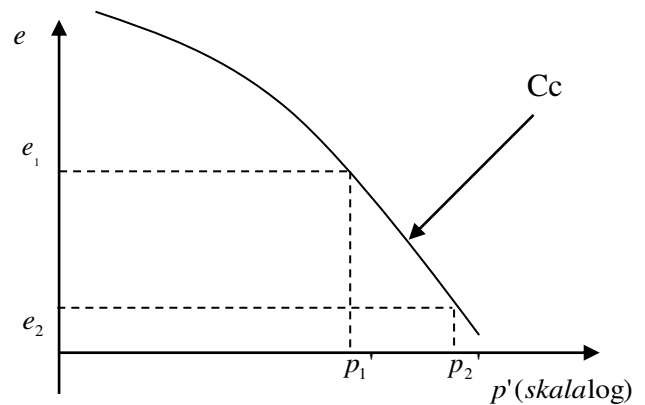
Gambar 1. Indeks Pemampatan C_c
