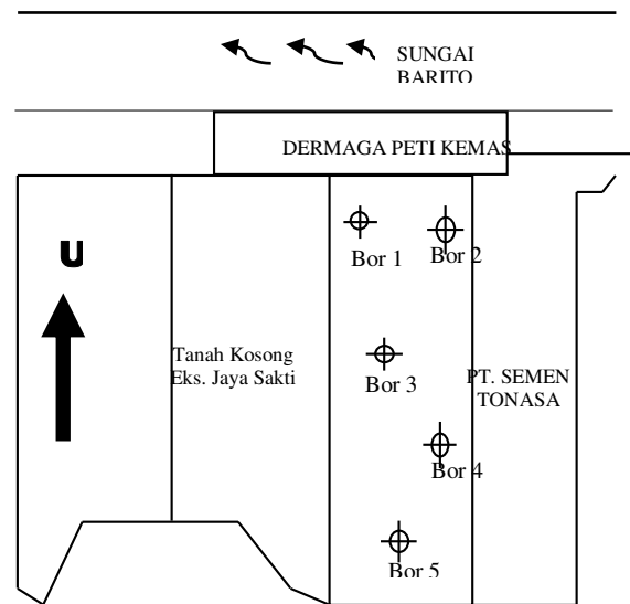
Gambar 4 Lay out titik bor
