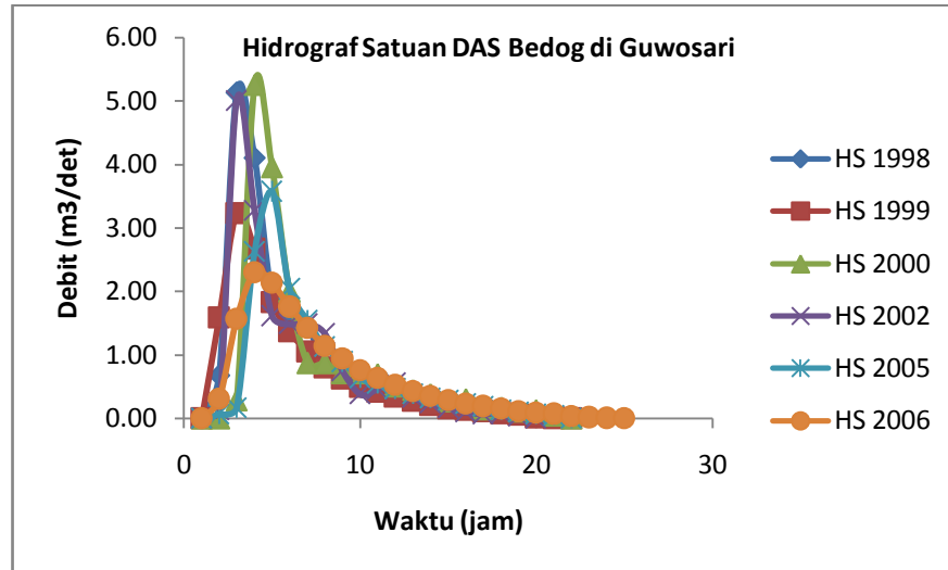
Gambar 6. Hidrograf satuan setiap kejadian banjir terpilih DAS Bedog di Guwosari
