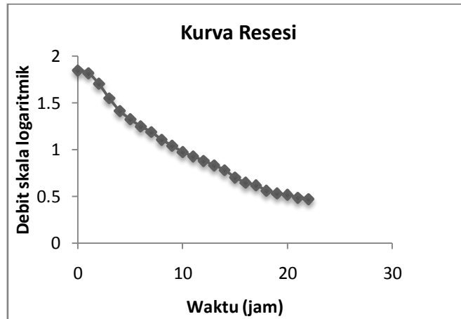
Gambar 4. Kurva debit semi logaritmik untuk mendapatkansisi resesi
