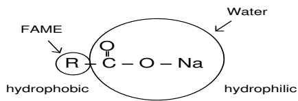
Gambar 6. Molekul sabun
