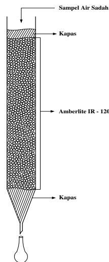
Gambar. 1 Rangkaian Alat Kromatografi Kolom Sederhana
