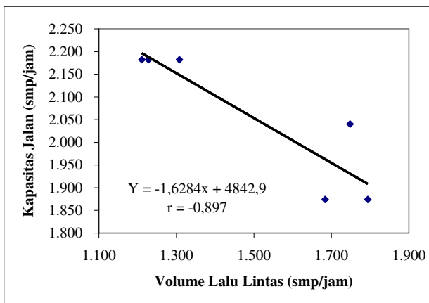
Gambar 1. Hubungan Volume Lalu Lintas dengan Kapasitas Jalan Dari Arah Jembatan Merdeka ke Pasar Kuripan.
