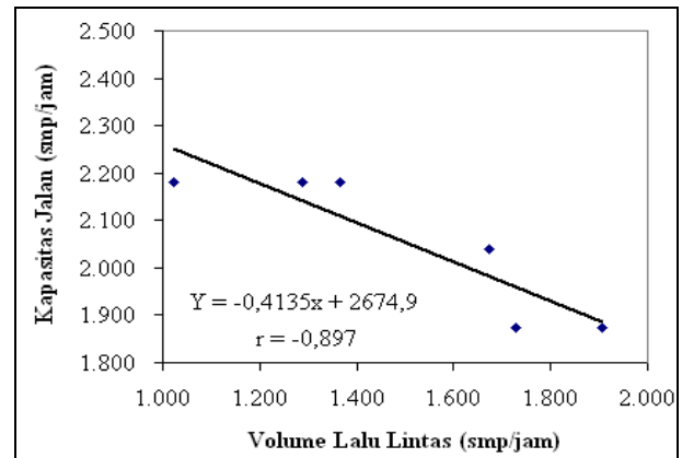
Gambar 2. Hubungan Volume Lalu Lintas dengan Kapasitas Jalan Dari Arah Pasar Kuripan ke Jembatan Merdeka.
