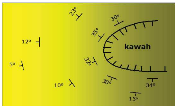
Gambar 11. Sketsa jurus dan kemiringan awal perlapisan batuan gunungapi yang berpola konsentris dan melandai menjauhi kawah gunung api.
