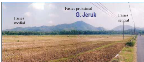
Gambar 5. Morfologi lereng-kaki selatan Gunung Jeruk, yang diperkirakan sebagai fasies sentral-proksimal-medial gunung api Tersier Ijo-Kukusan di Pegunungan Kulonprogo, Yogyakarta. Puncak Gunung Ijo dan Gunung Kukusan terletak di sebelah kanan gambar.
