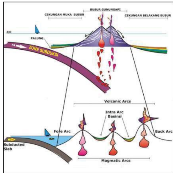
Gambar 12. Cekungan di dalam busur gunung api ( intra-arc basins ), yang terbentuk di antara kerucut gunung api di dalam zone busur gunung api. Dibanding dengan cekungan busur muka ( fore arc basin ) dan cekungan busur belakang ( back arc basin ), maka cekungan di dalam busur gunung api relatif lebih kecil tetapi banyak; proses sedimentasi, aktivitas tektonika, magmatisme dan vulkanisme sangat aktif, melibatkan berbagai kondisi lingkungan pengendapan, terutama mulai dari laut dangkal sampai darat kering (Bronto dr., 2006).
