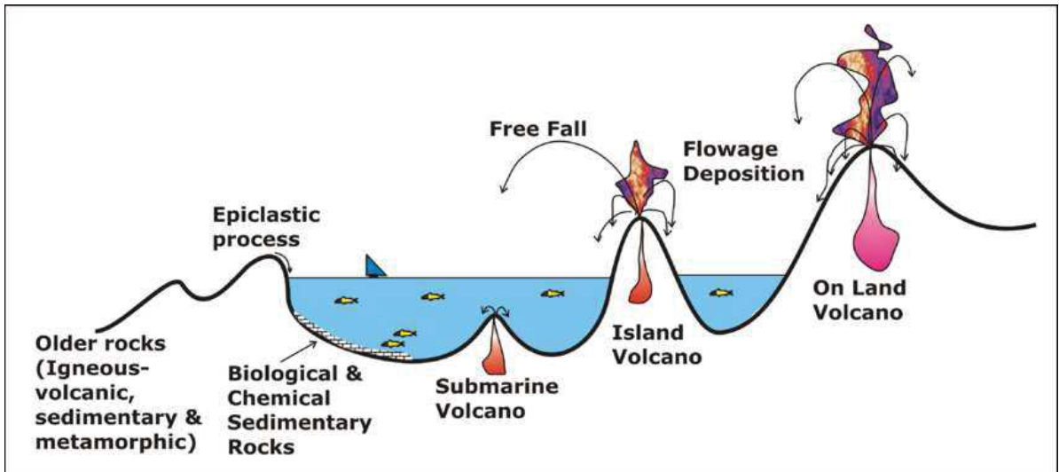
Gambar 13. Sedimentasi di dalam Cekungan Salome, sebagai bagian dari cekungan di dalam busur gunung api. Sumber material berasal dari pengerjaan ulang batuan tua (proses epiklastika, membentuk batuan silisiklastika), proses biologi dan kimia yang membentuk batuan sedimen klastika dan non klastika, serta kegiatan gunung api bawah laut ( submarine volcano ), pulau gunung api ( island volcano ) dan gunung api di darat ( on land volcano ) yang membentuk batuan beku koheren dan batuan klastika gunung api.
