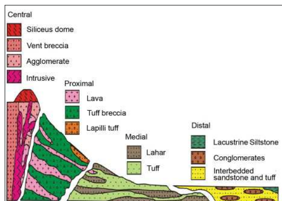
Gambar 1. Pembagian fasies gunung api menjadi fasies sentral, fasies proksimal, fasies medial, dan fasies distal beserta komposisi batuan penyusunnya (Bogie & Mackenzie, 1998).
