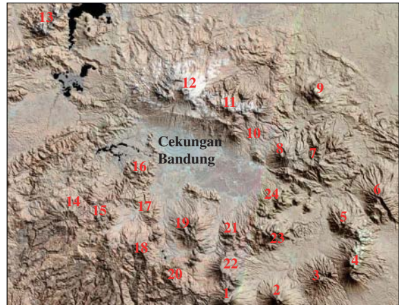
Gambar 6. Citra landsat daerah Bandung dan sekitarnya yang memperlihatkan bentuk bentang alam kerucut gunung api muda (misal nomor 1, 2, 4, 8, dan 9) sampai tua (nomor 3, 7, 11, 13, 16, dan 18). Gunung api muda dicirikan oleh bentuk kerucut yang relatif masih utuh dengan pola aliran memancar dari pusat erupsi. Semakin tua relief gunung apinya semakin kasar sebagai akibat erosi yang semakin lanjut dan aliran sungai cenderung ke pola mendaun. Urutan nama gunung api di dalam teks.
