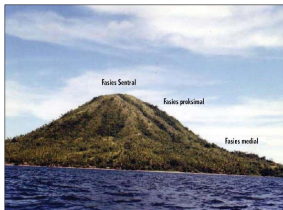
Gambar 3. Pulau Maitara di daerah Ternate, Maluku Utara sebagai salah satu pulau gunung api Kuartar di mana fasies distalnya berada di bawah muka air laut.
