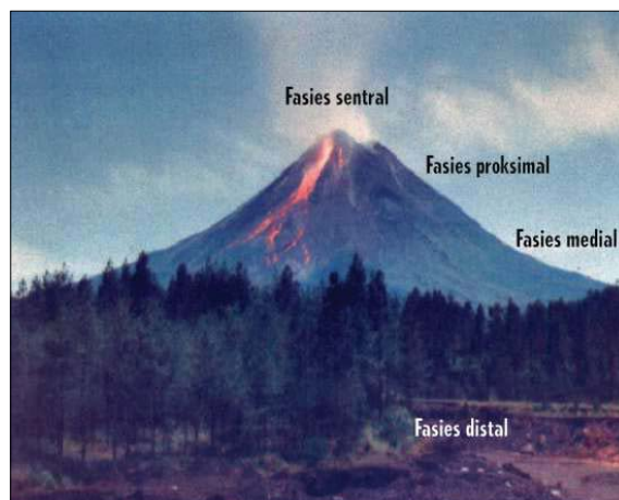
Gambar 2. Pembagian fasies gunung api pada gunung api aktif masa kini seperti halnya di kerucut komposit Gunung Merapi, Jawa Tengah. Fasies sentral terletak di bagian puncak atau pusat erupsi, fasies proksimal pada lereng atas dan fasies medial di lereng bawah. Fasies distal terletak di kaki dan dataran di sekeliling gunung api, di antaranya dataran di latar depan gunung api.
