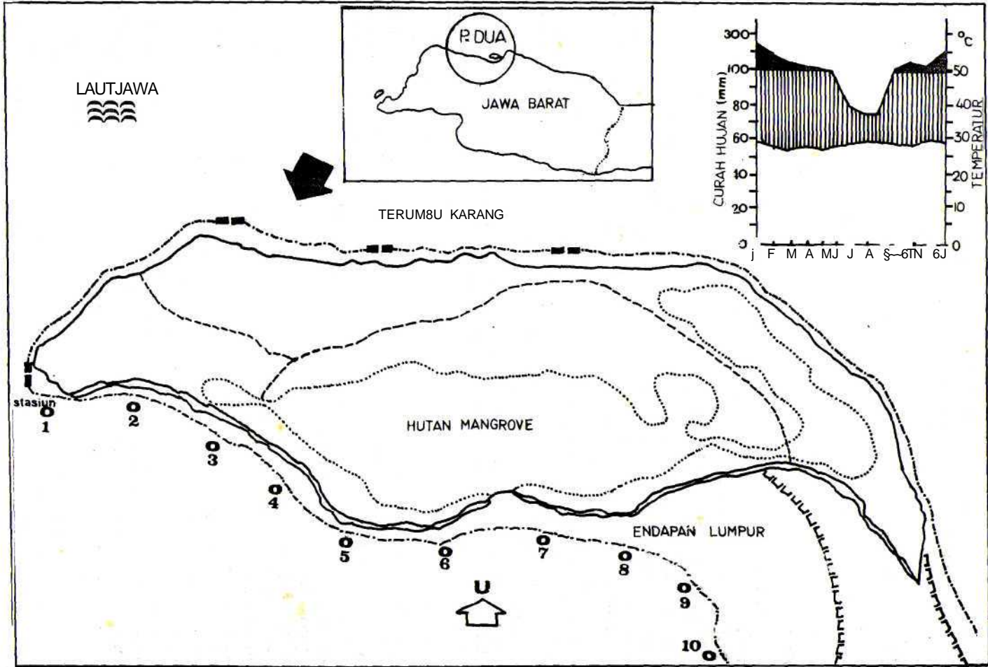
Gambar 1. Peta P. Dua, Banten beserta stasiun pengamatan.
