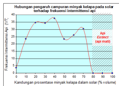
Gambar 5. Hubungan antara pengaruh campuran minyak kelapa pada bahan bakar solar terhadap frekuensi intermittensi api
