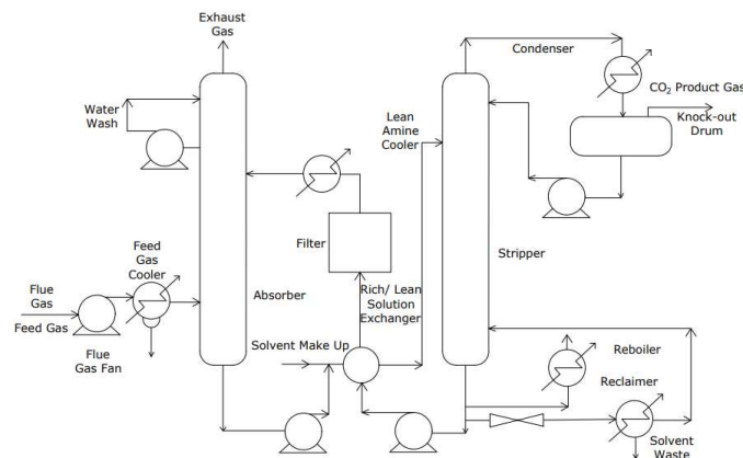
Gambar 3. 1 Skema Operasi CO 2 Capture
