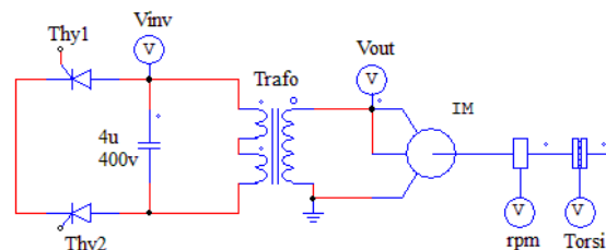
Gambar 10. Rangkaian inverter menggunakan dua buah thyristor dengan output motor induksi 1 fasa.
