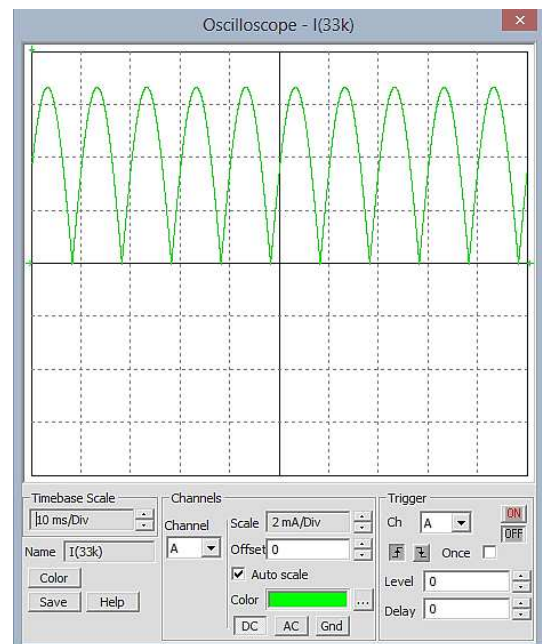
Gambar 6. Bentuk gelombang Idc pada resistor 33KΩ dari Osiloskop PSIM.
