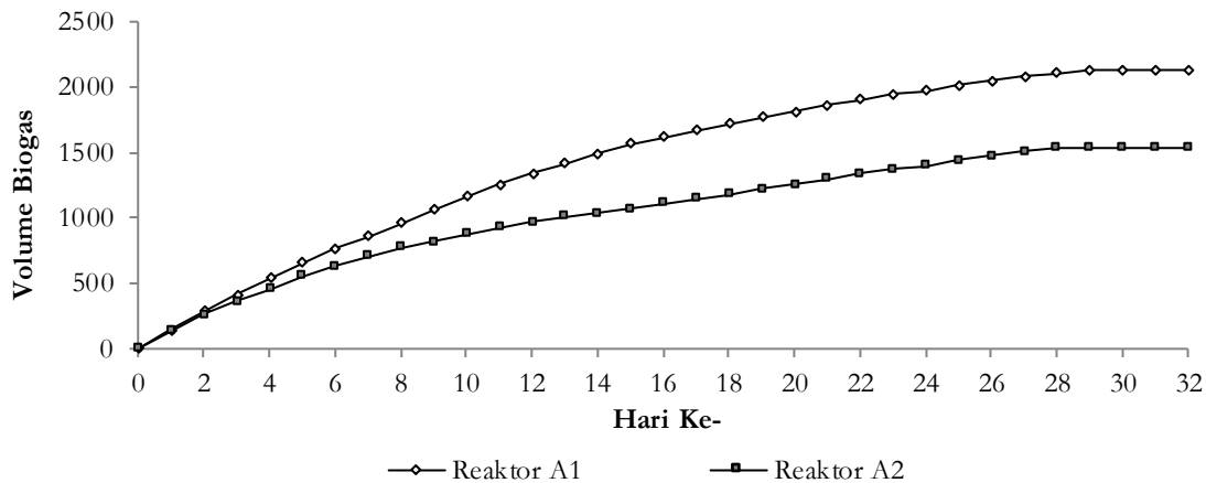
Gambar 6. Grafik akumulasi volume produksi biogas
