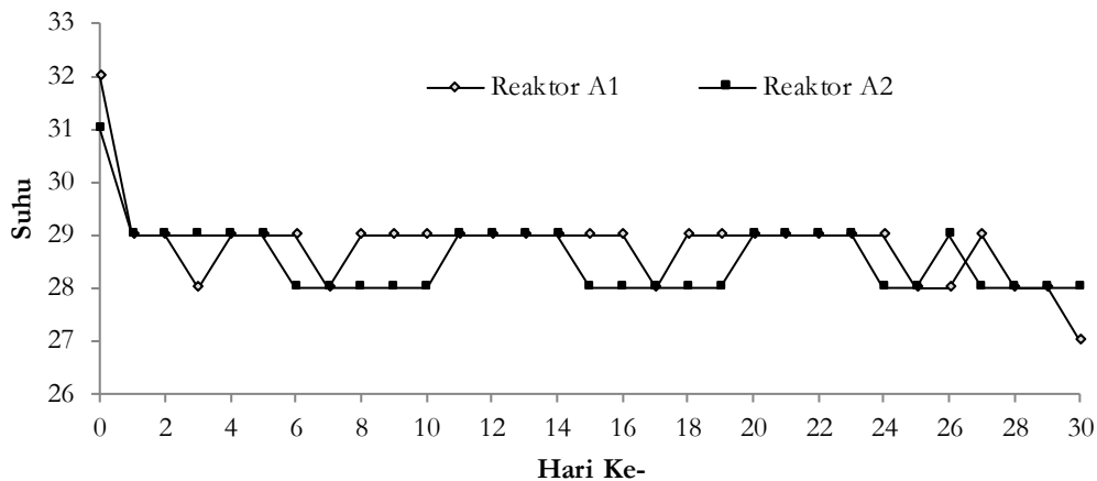
Gambar 1. Suhu pada slurry
