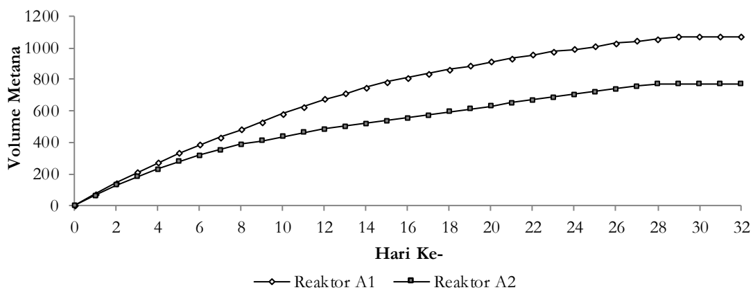
Gambar 7. Grafik akumulasi volume produksi metana
