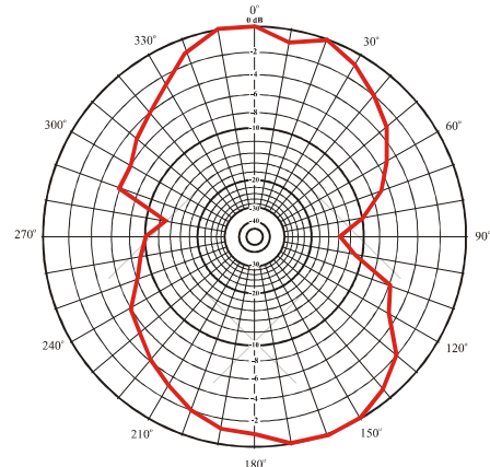
Gambar 8 Bentuk Polarisasi Antena Mikrostrip Array
