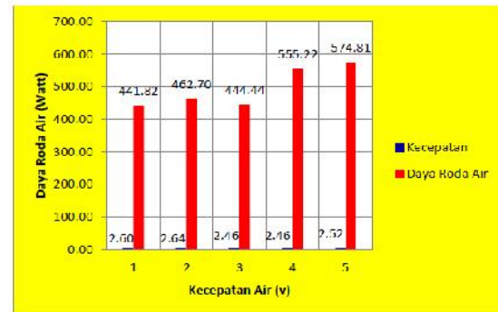
Gambar 9. Hubungan kecepatan air dengan daya roda air
