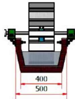
Gambar 2. Tampak depan saluran
