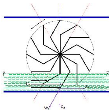
Gambar 11. Analisa kecepatan relatif air terhadap sudu pada sisi keluar
