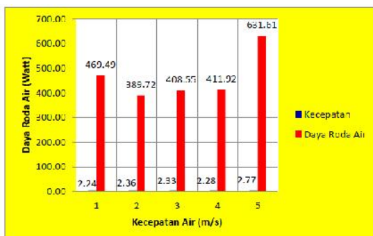
Gambar 8. Hubungan kecepatan air dengan daya roda air
