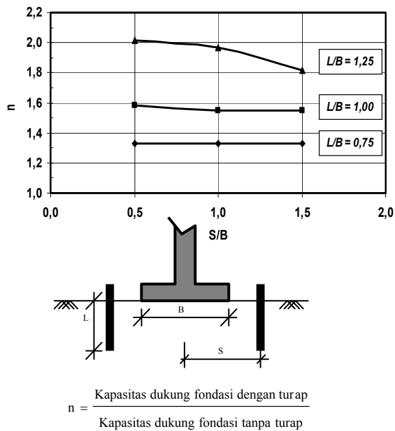
Gambar 7 Hubungan antara letak turap dan kapasitas dukung fondasi dengan turap.
