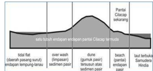
Gambar 1. Satu sekuen tubuh endapan Pantai Cilacap.
