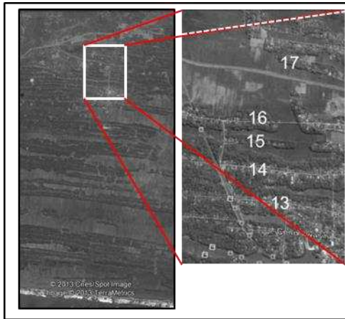
Gambar 8. Interpretasi garis pantai purba bagian tengah daerah penelitian.
