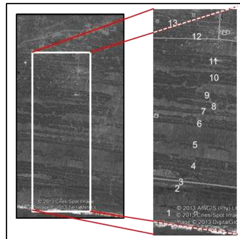
Gambar 7. Interpretasi garis pantai yang ada dan pernah ada di selatan daerah penelitian.
