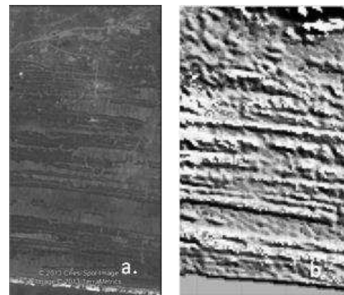
Gambar 2. Kenampakan daerah penelitian dalam citra Google Earth (a), dan SRTM (b).
