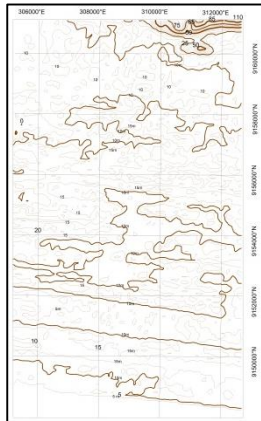
Gambar 3. Peta topografi daerah penelitian.
