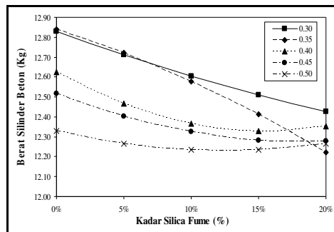
Gambar 2. Grafik berat sampel silinder beton dengan variasi kadar silica fume dan fas
