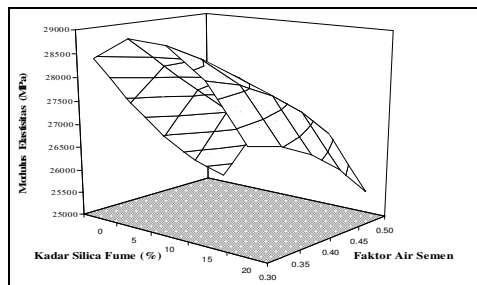
Gambar 3. Grafik hubungan antara kadar silica fume dan faktor air semen (fas) terhadap modulus elastisitas beton
