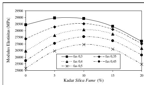
Gambar 4. Grafik hubungan antara silica fume dan modulus elastisitas beton
