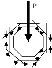
Gambar 4 Aksi Serat bersama Pasta Semen.
