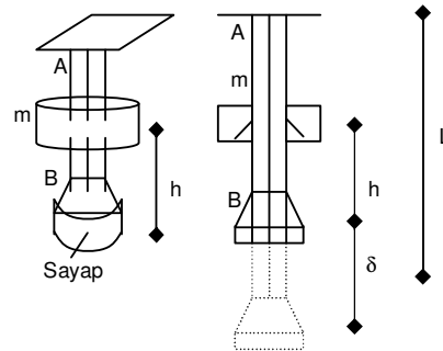
Gambar 6 Beban kejut batang prismatik akibat jatuhnya benda bermassa m.
