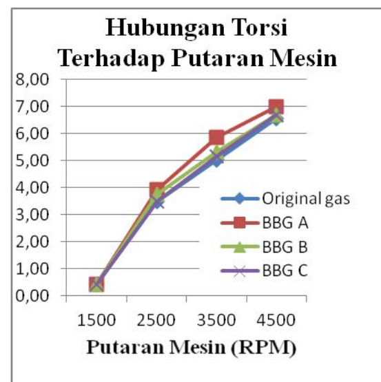
Gambar 2. Hubungan torsi terhadap putaran mesin
