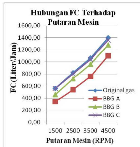
Gambar 4. Hubungan FC terhadap putaran mesin
