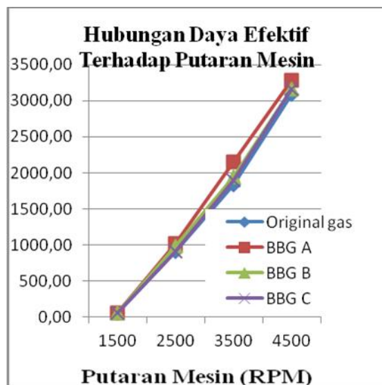
Gambar 3. Hubungan daya efektif terhadap putaran mesin
