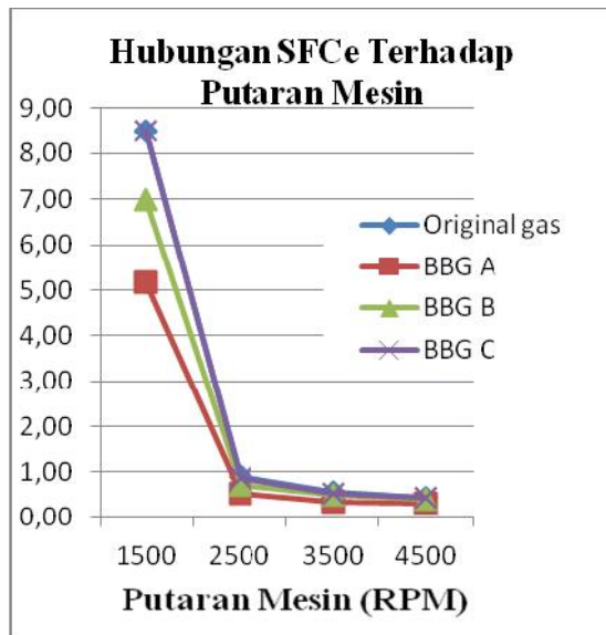
Gambar 5. Hubungan SFCe terhadap putaran mesin
