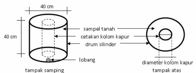
Gambar 3 Bak pengujian.
