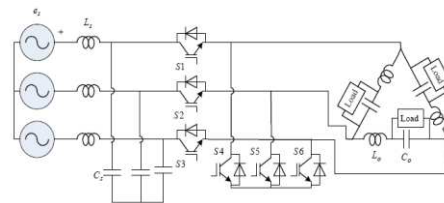
Gambar 3. Rangkaian AC Chopper 3-fasa
