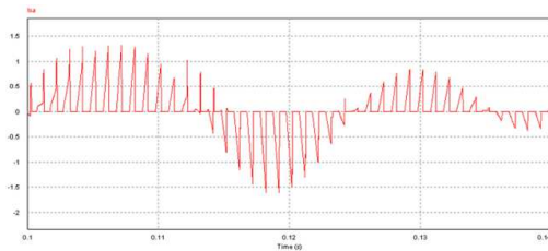
Gambar 11. Gelombang Output Beban Motor Induksi 3-Fasa
