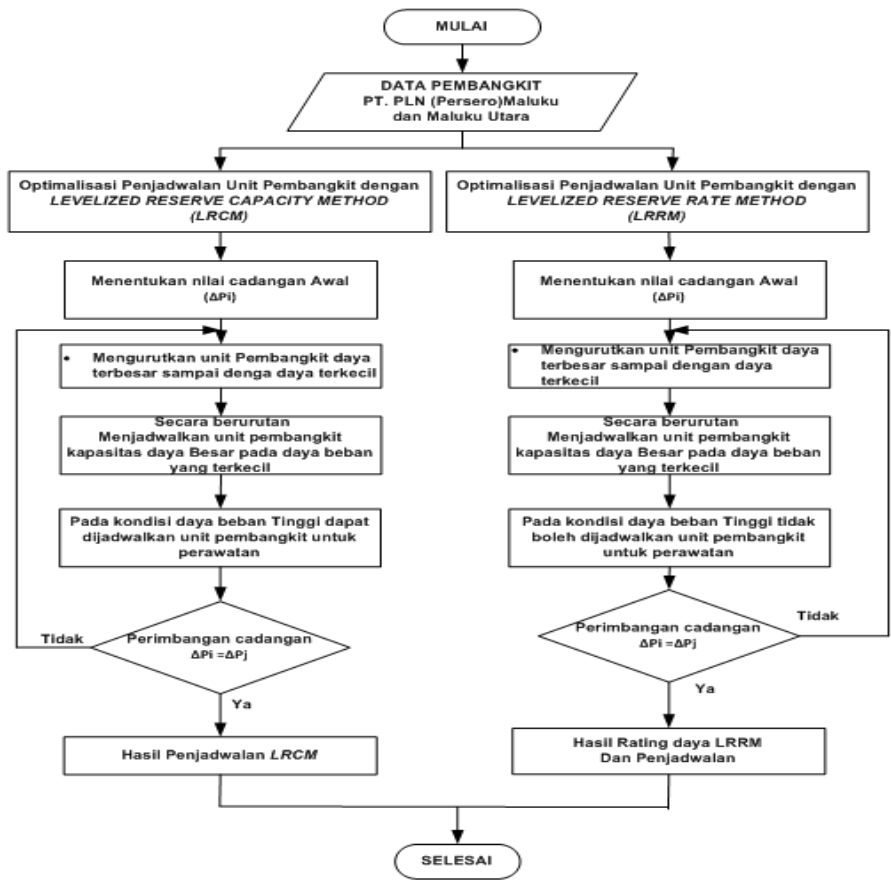
Gambar 1. Diagram alir metodologi penelitian
