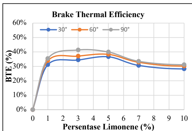
Gambar 5 Pengaruh prosentase limonen dalam bahan bakar terhadap termal efisiensi motor bensin
