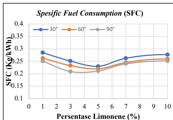
Gambar 4 Pengaruh prosentase limonen dalam bahan bakar terhadap konsumsi bahan bakar motor bensin
