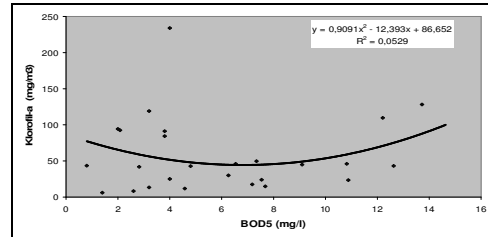
Gambar 3. Grafik hubungan antara BOD 5 dengan klorofil-a
