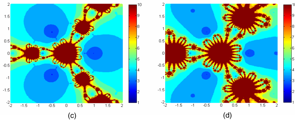
Gambar 4. Basin attraktor f_7 = x^3 - 1 (a) AM (b) GM (c) PSM (d) HM
