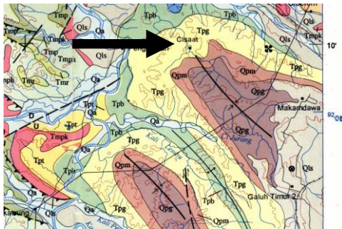
Gambar 4. Peta geologi tempat pengambilan sampel lintasan sungai Cisaat Menurut Kastowo dan Suwarna (1996)
