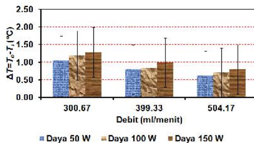
Gambar 4. Pengaruh debit aliran dan daya panas terhadap T .
