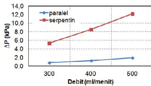
Gambar 9. Hubungan P dengan debit debit 300, 400 dan 500 \text{cm}^3/\text{menit} pada pipa paralel dan serpentin.
