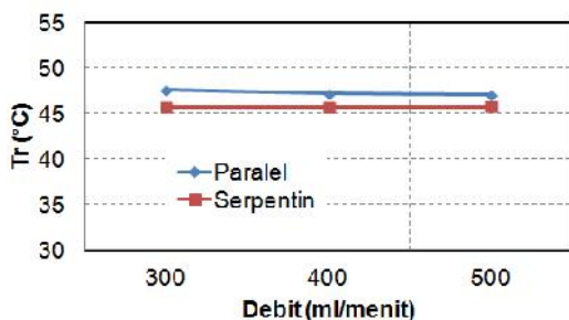
Gambar 6. Hubungan T_r dengan debit debit 300, 400 dan 500 \text{cm}^3/\text{menit} pada pipa paralel dan serpentin dengan daya 50 W.
