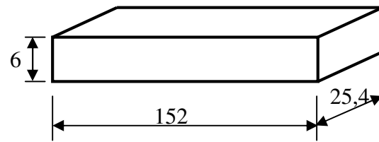
Gambar 4. Spesimen uji bending ASTM D 790
