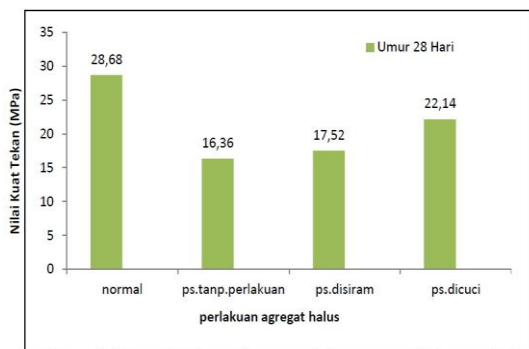
Gambar 4. Nilai kuat tekan beton dengan perlakuan agregat halus yang berbeda pada umur 28 hari
