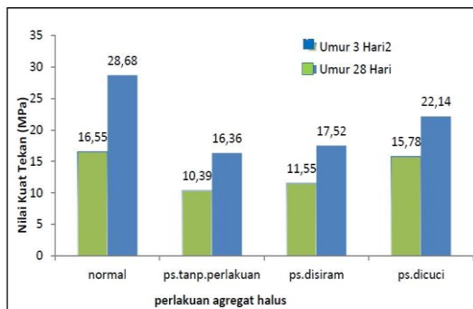
Gambar 5. Gabungan nilai kuat tekan beton dengan perlakuan agregat halus yang berbeda pada umur 3 hari dan umur 28 hari
