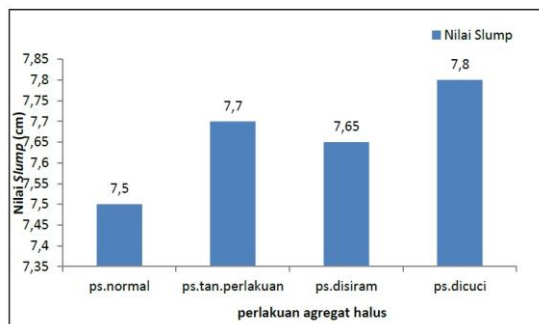
Gambar 2. Nilai slump dengan perlakuan agregat halus yang berbeda
