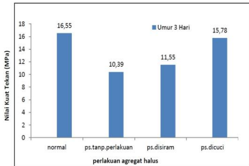
Gambar 3. Nilai kuat tekan beton dengan perlakuan agregat halus yang berbeda pada umur 3 hari
