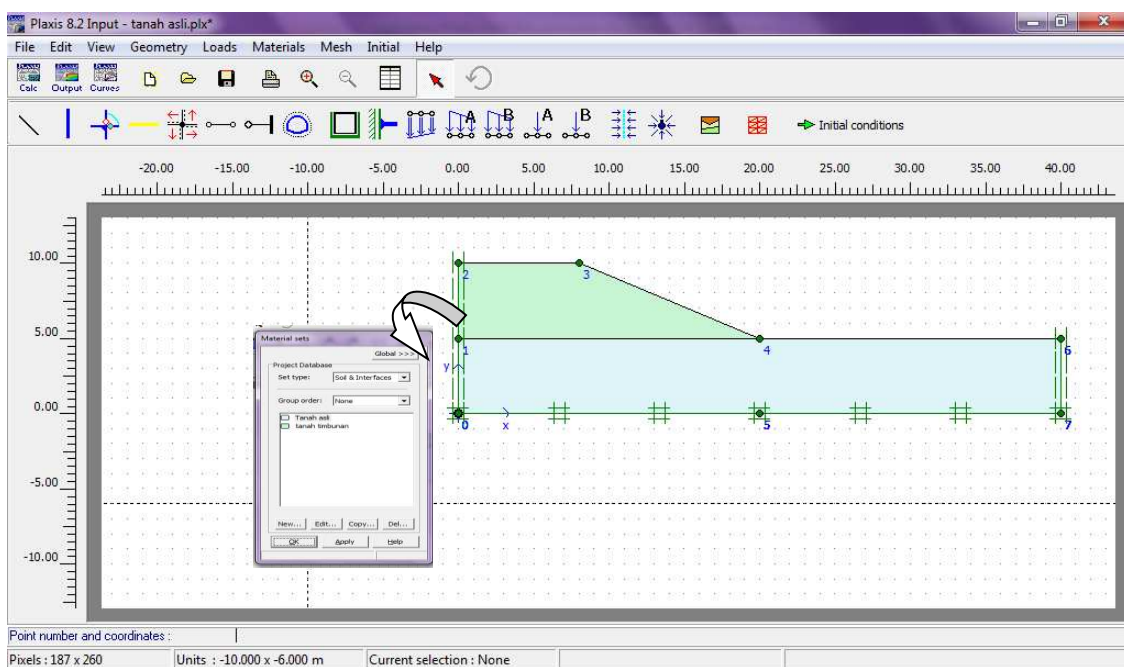
Gambar 2. Input Geometri
