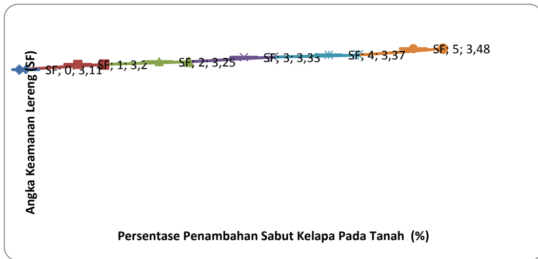
Gambar 6. Grafik Angka Kemananan Lereng Terhadap Penambahan Sabut Kelapa Pada Tanah
