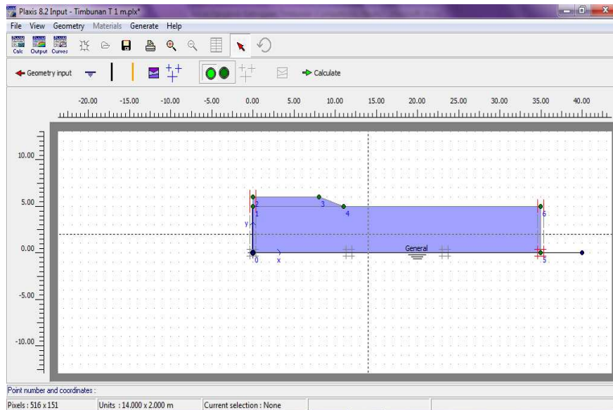
Gambar 5. Input standart fixities , pembebanan, jaringan lement ( mesh ), ground water condition pada lapisan tanah
