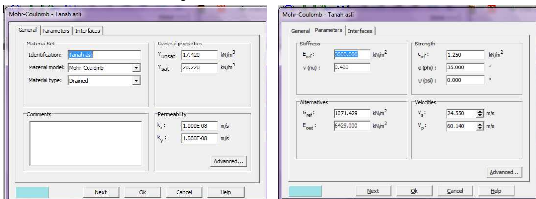
Gambar 3. Input Parameter Tanah Asli
