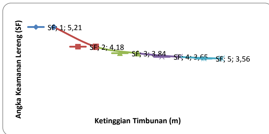
Gambar 8. Grafik Angka Kemananan Lereng Terhadap Ketinggian Timbunan
