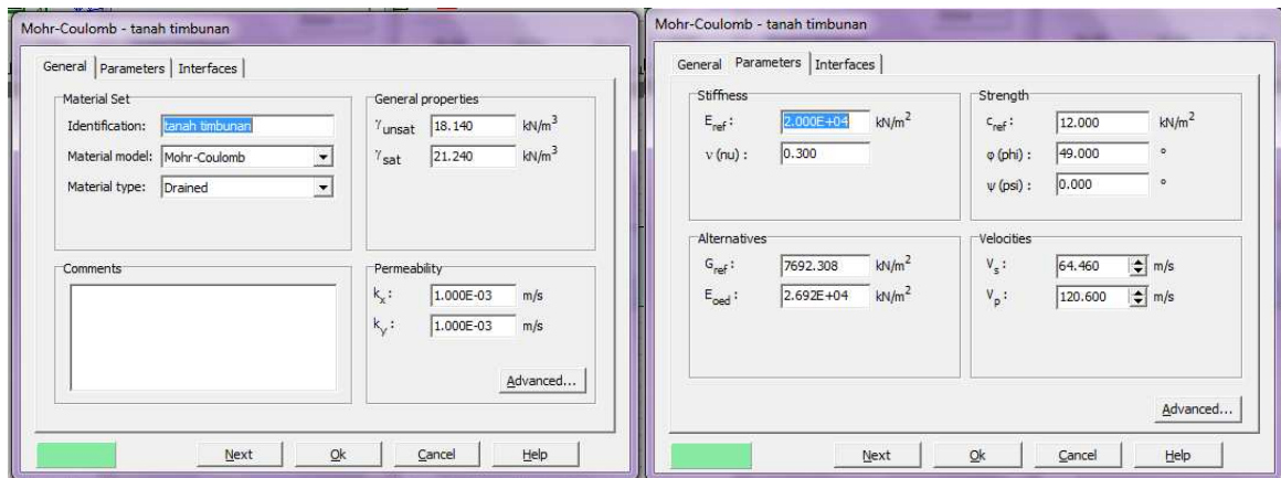
Gambar 4. Input Parameter Tanah Timbunan
