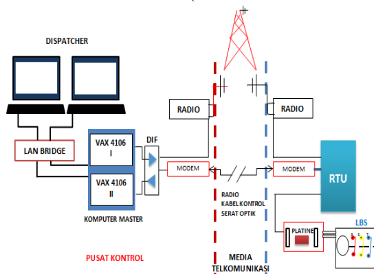
Gambar 1. Bagian Komponen SCADA
