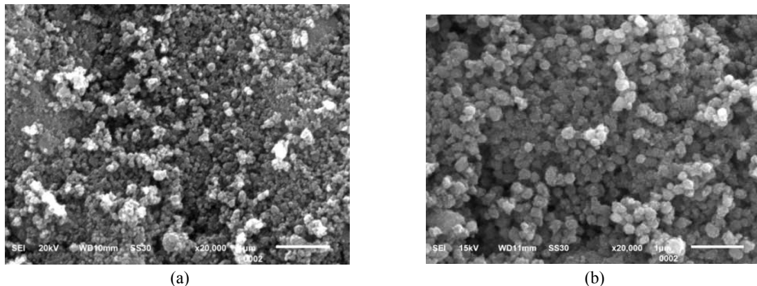
Gambar 2. Morfologi TiO 2 Nanopartikel konsentrasi 0,3M dengan penambahan templat kanji (a) tanpa penambahan templat, dan (b) dengan templat kanji
