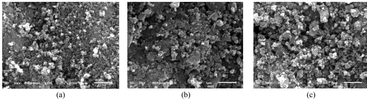
Gambar 1. Morfologi TiO 2 nanopartikel tanpa penambahan templat kanji konsentrasi (a) 0,3 M, (b) 0,5M dan (c) 1,0 M pada temperatur 500°C
