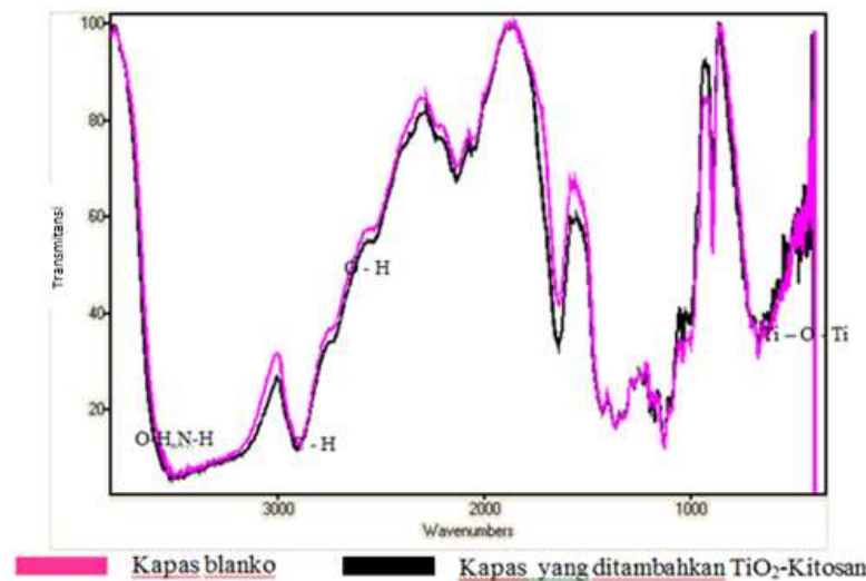
Gambar 5. Spektrum Kain yang Diberi Perlakuan \text{TiO}_2
