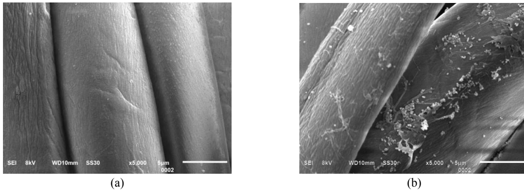
Gambar 4. Analisa Morfologi Kapas dengan Penambahan \text{TiO}_2 Nanopartikel Menggunakan SEM (a) Kapas yang tidak diberi perlakuan \text{TiO}_2 , (b) Kapas yang diberi perlakuan \text{TiO}_2
