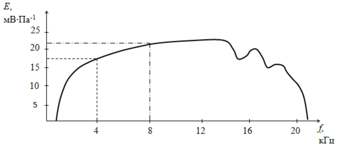
Рисунок 1 – Амплітудно-частотна характеристика мікрофона
