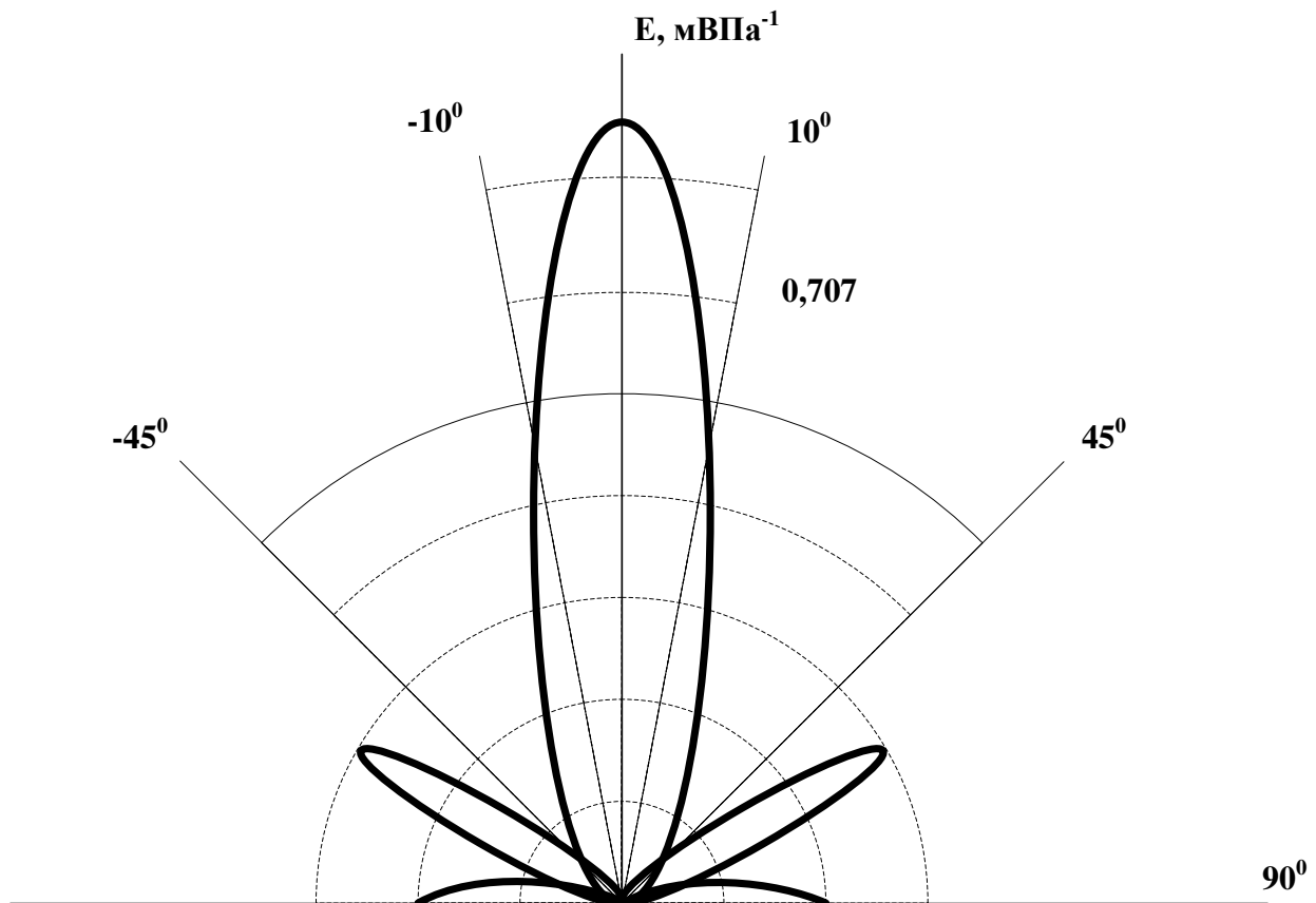
Рисунок 2 – Характеристика спрямованості мікрофона (в горизонтальній площині)
