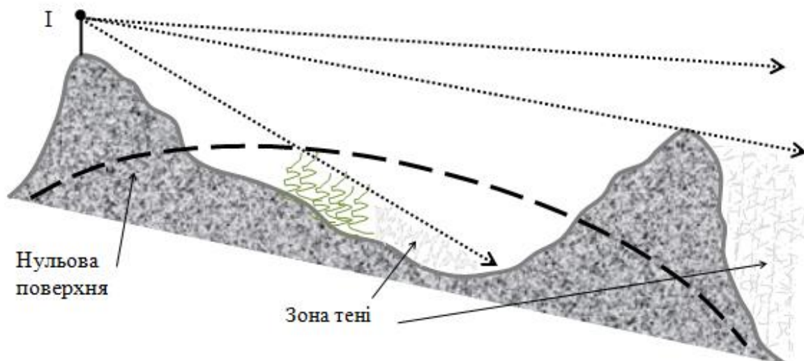
Рисунок 4 – Схема формування зон освітленості і зон тіні
