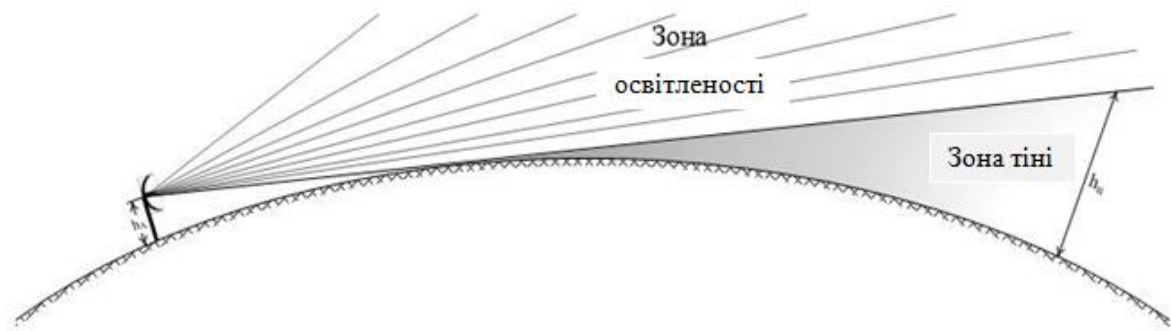
Рисунок 3 – Схема формування зон освітленості та тіні за рахунок скривлення земної поверхні
