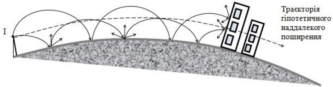
Рисунок 6 – Схема перешкоди наддалеке поширення звуку житловим масивом
