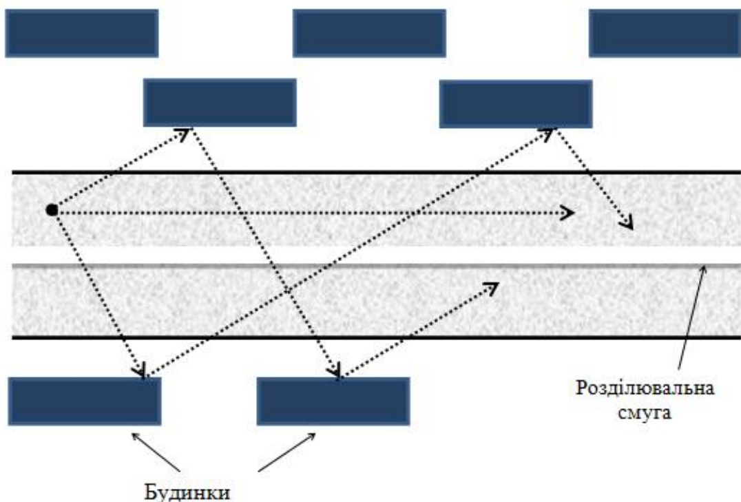
Рисунок 7 – Схема каналізації акустичної енергії в житловому масиві
