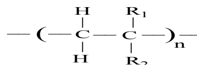
Fig. 2. Degrading polymer.
