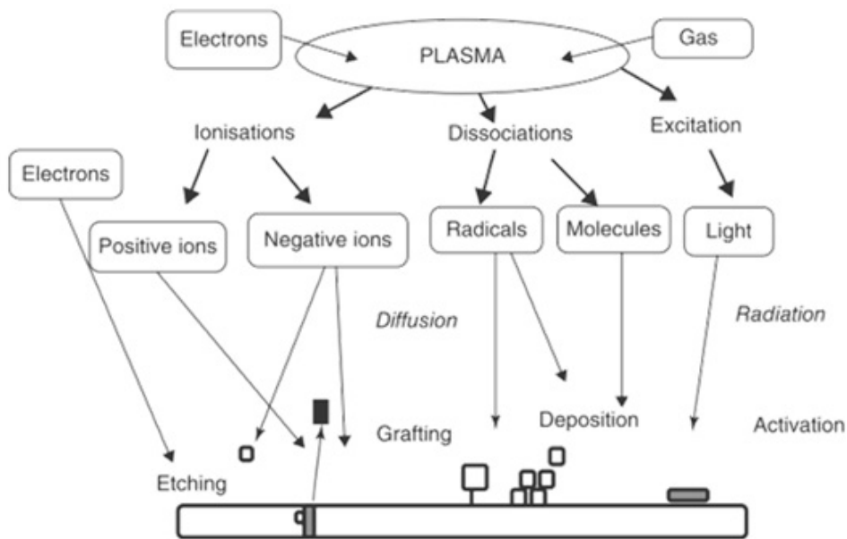
Gambar 2. Ilustrasi proses etsa permukaan bahan polimer menggunakan proses plasma 13
