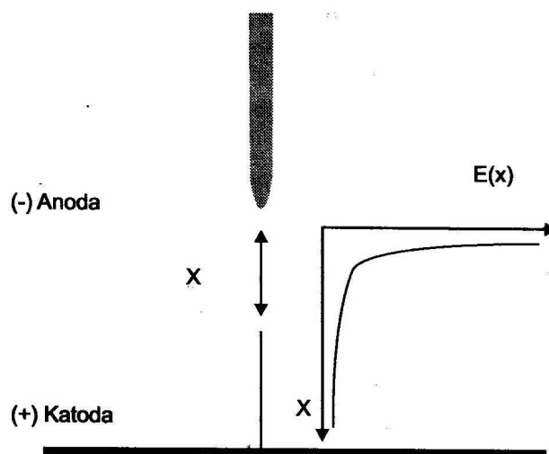
Gambar 4. Kuat medan listrik sebagai fungsi jarak. 9
