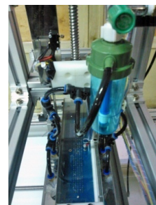
d. Elektrodapada plasma chamber
