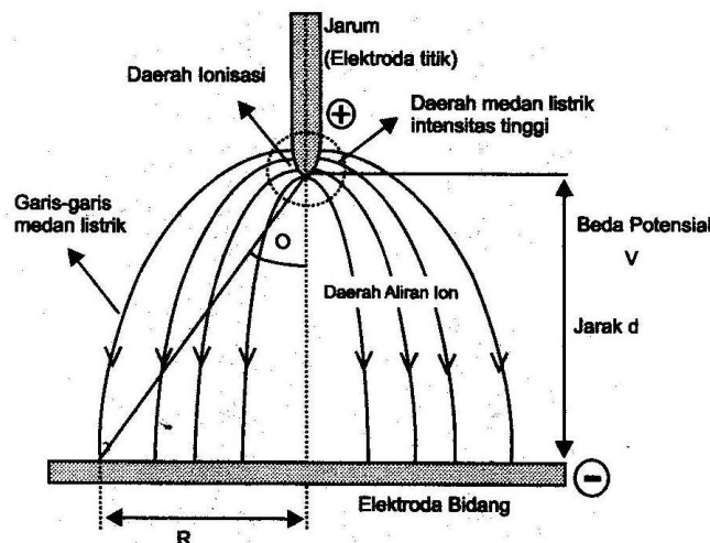
Gambar 3. Daerah ionisasi dan aliran pada lucutan pijar korona. 9
