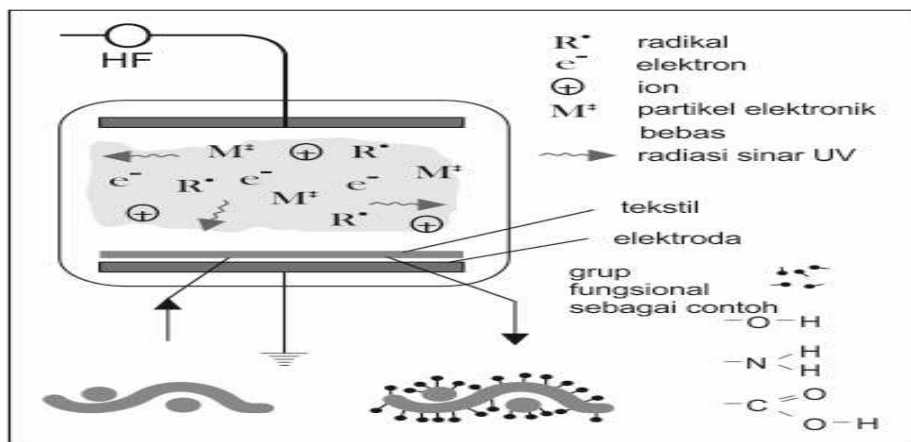
Gambar 1. Ilustrasi proses plasma pada bahan kain 4
